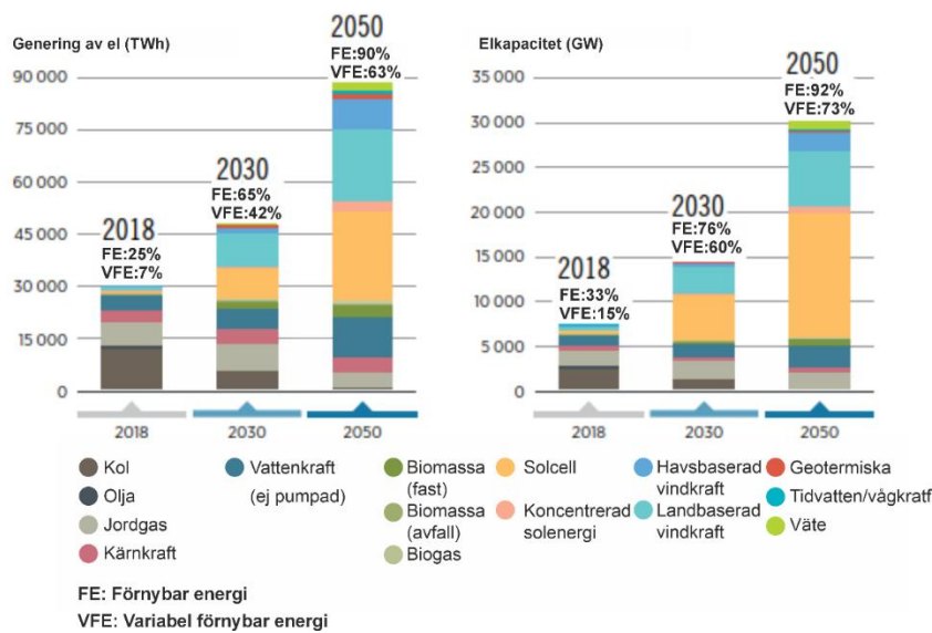
Bild 4.1 Total elproduktion och kapacitet för elproduktionskällor som krävs enligt 1,5°C-målet 2018, 2030 och 2050 (källa: IRENA 2022, bild 2.3.)
